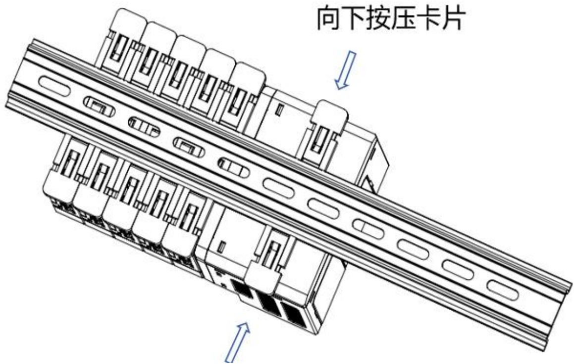
图 2-7 主机导轨安装示意图
