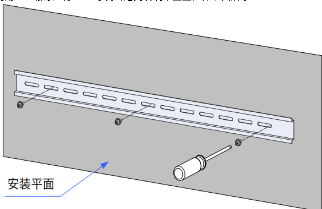
图 2-6 DIN 导轨安装示意图
