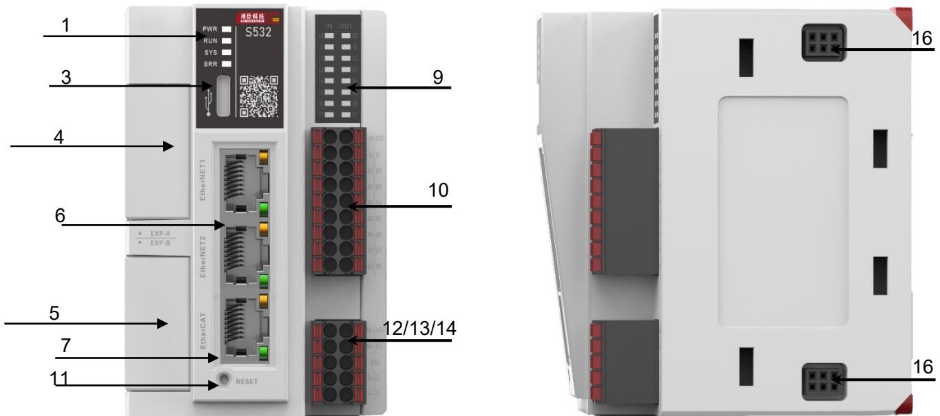
图1-2: S508-0808TN外部接线图
