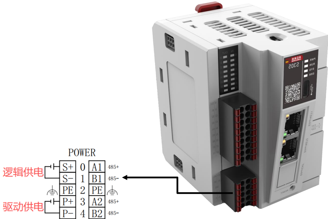
图1-3: S508-0808TN外部接线图
