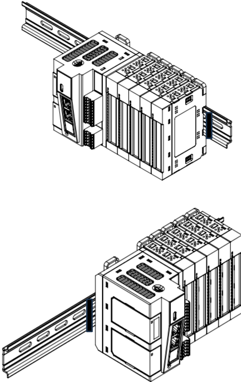
图：2-10 模块组装示意图
