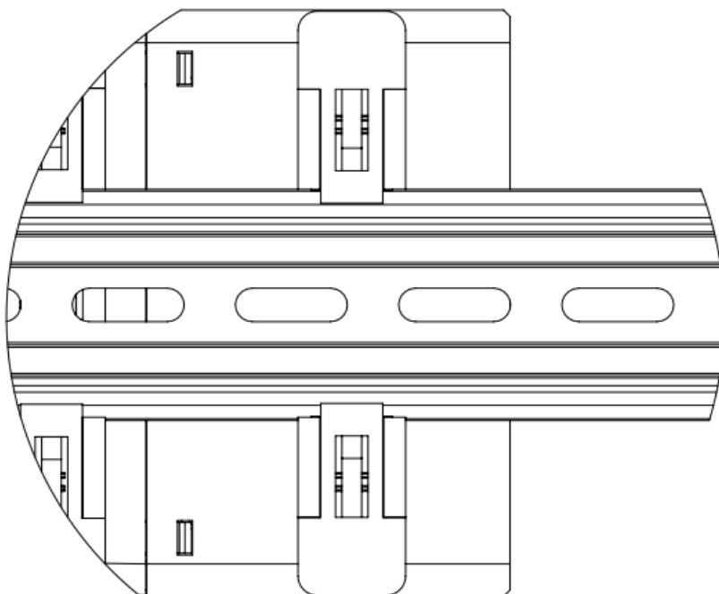
图 2-8 背面卡扣示意图
