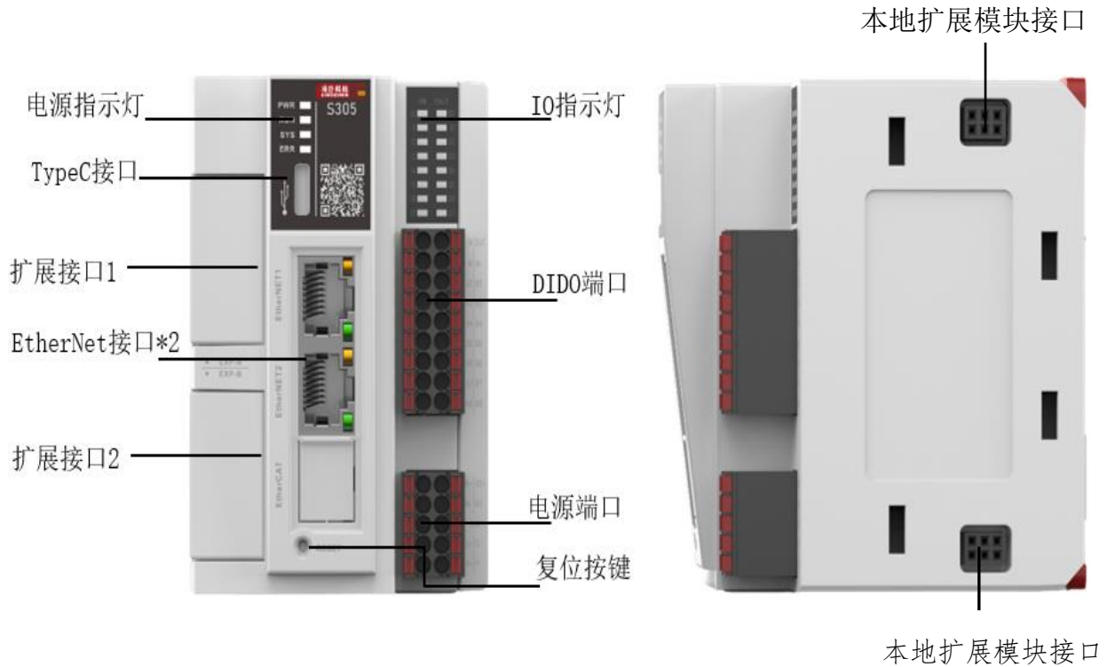
图1-1： S305-0808TN扩展模块接口
