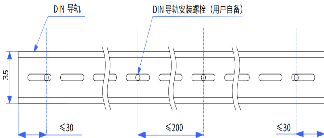
图 2-5 DIN 导轨安装螺栓位置要求 (单位: mm)
