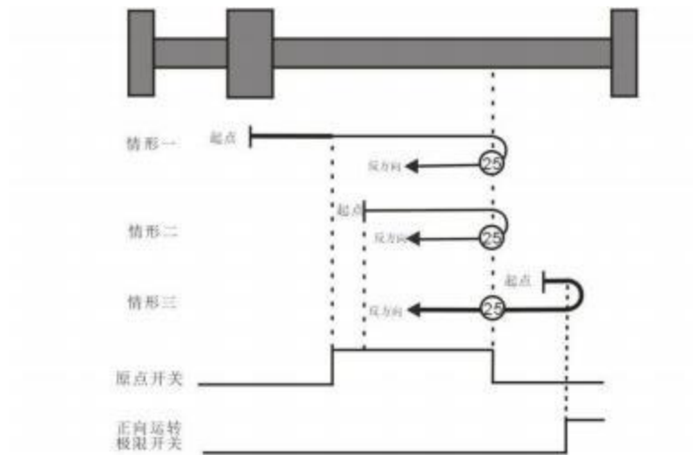
取决于原点开关、正向运转极限开关的原点回零，上图中的表示 \textcircled{25} 原点回零模式25
