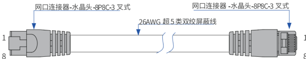
图4-18 EtherCAT网线制作要求
