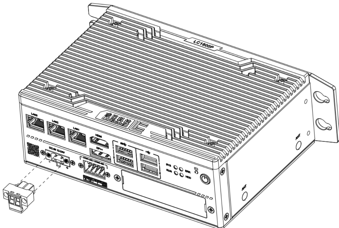
图 4-5 电源输入端子接线示意图
