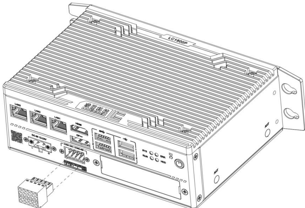
图4-6 用户端子接线示意图
