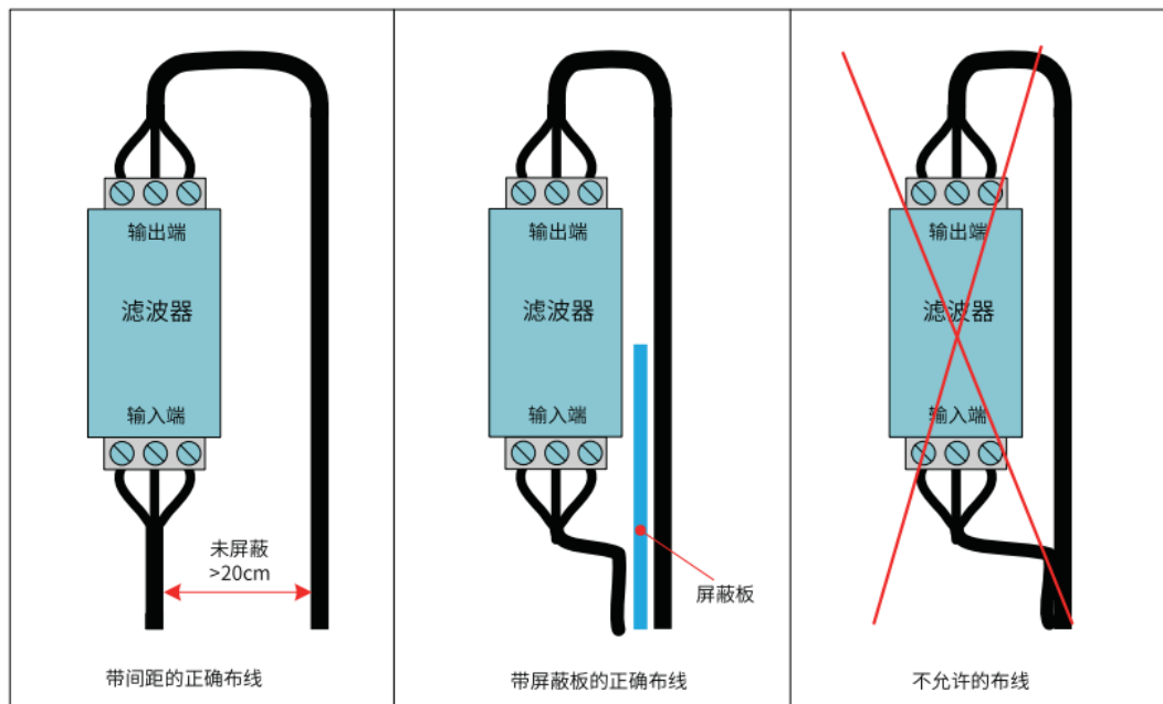
图 4-4 电源滤波器的安装示意图
