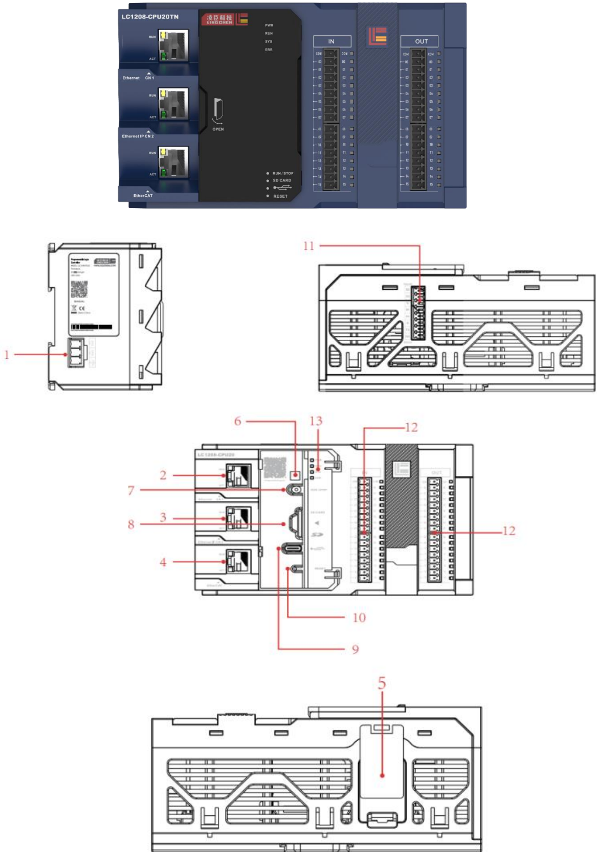
CPU 模块外部接口示意图
