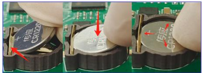
安装电池
