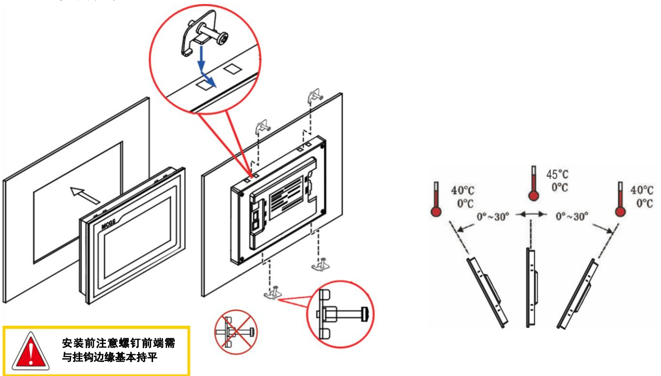
挂钩安装
